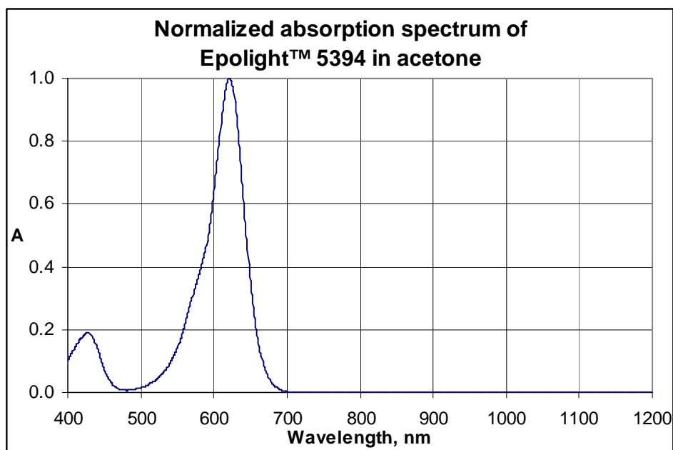
Epilight™ 5394 在丙酮中的标准化吸收光谱
