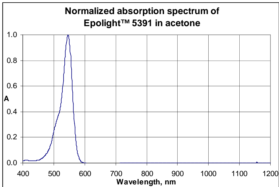
Epilight™ 5391 在丙酮中的标准化吸收光谱
